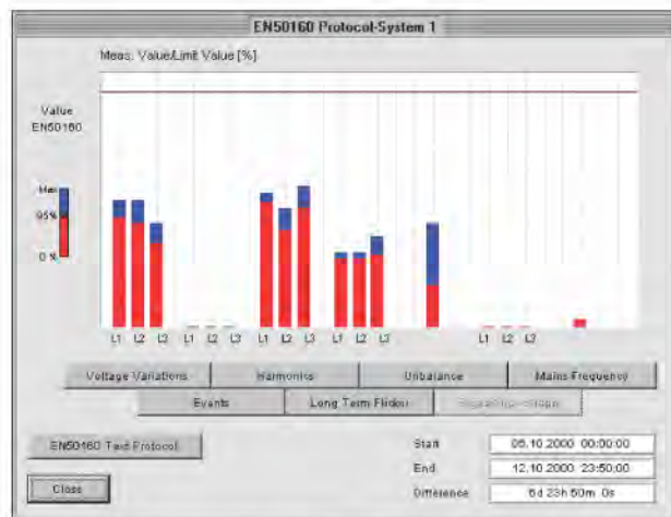
빠른 전력 품질 평가 - EN50160 국제 전력 품질 표준에 따라서 한 개의 dashboard에서 7개의 전력 품질 파라미터의 요약을 보여줍니다.
