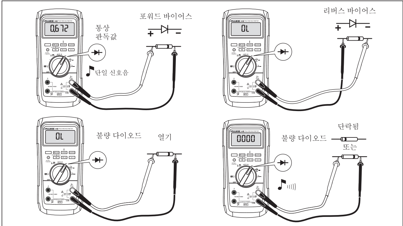
그림 7. 다이오드 테스트
